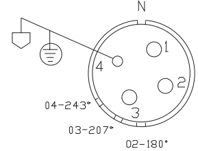
CN-06-22/CN-06-322 4 #10 Contacts
