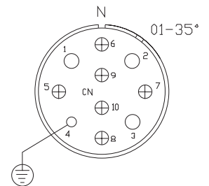
CN-08-376 6 #12 & 4 #10 Contacts
